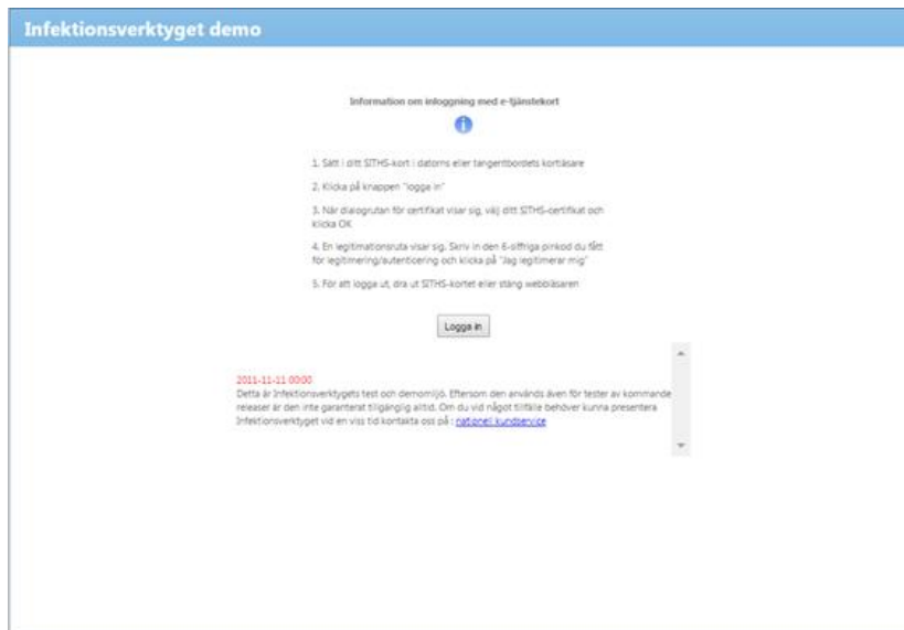
Figur 1 Rapportverkygets inloggningssida
