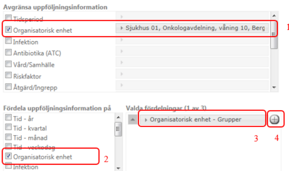
Figur 5 Skapa grupper.
