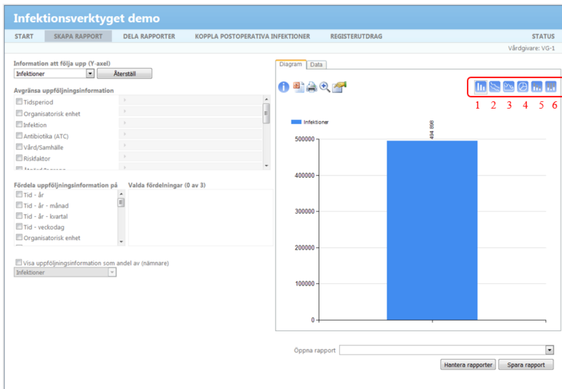
Figur 7 Tillgängliga diagramtyper
