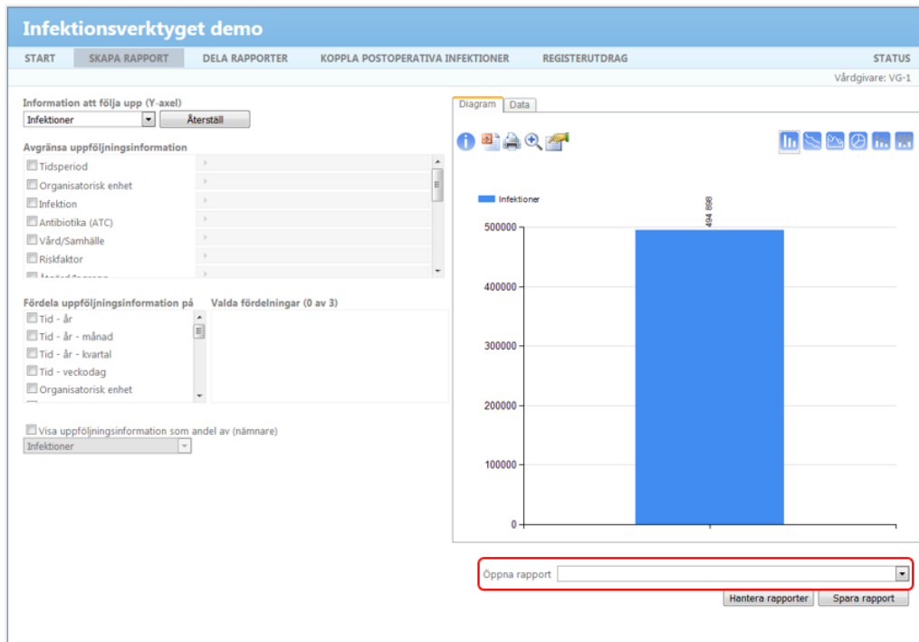
Figur 14 Öppna rapport.
