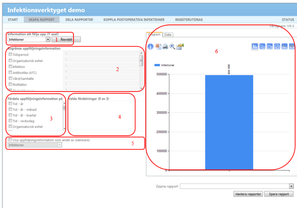
Figur 4 Skapa rapport
