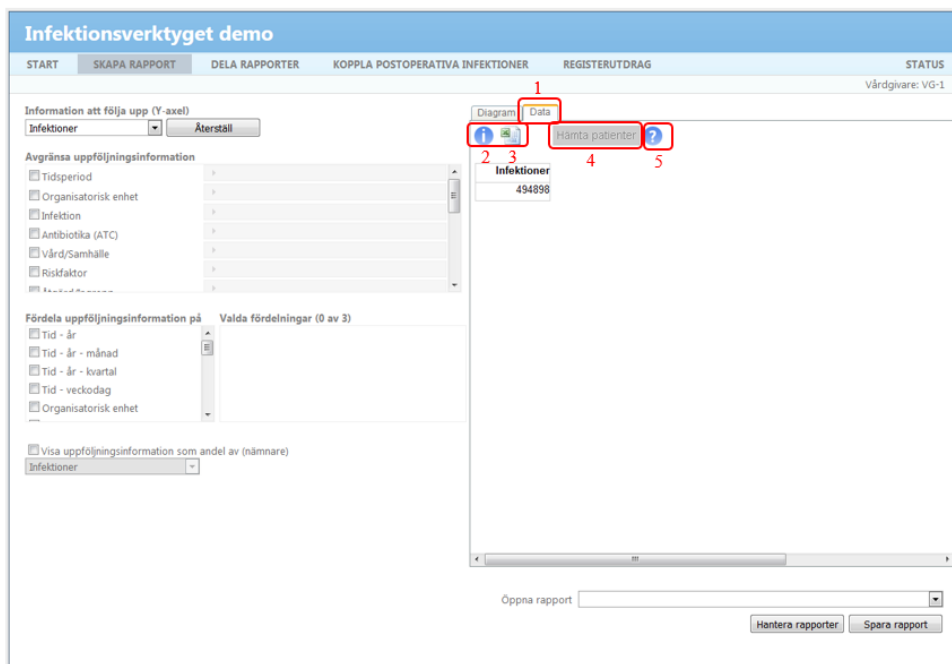
Figur 17 Fliken data.
