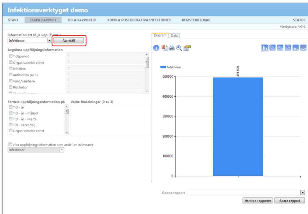
Figur 13 Återställ.
