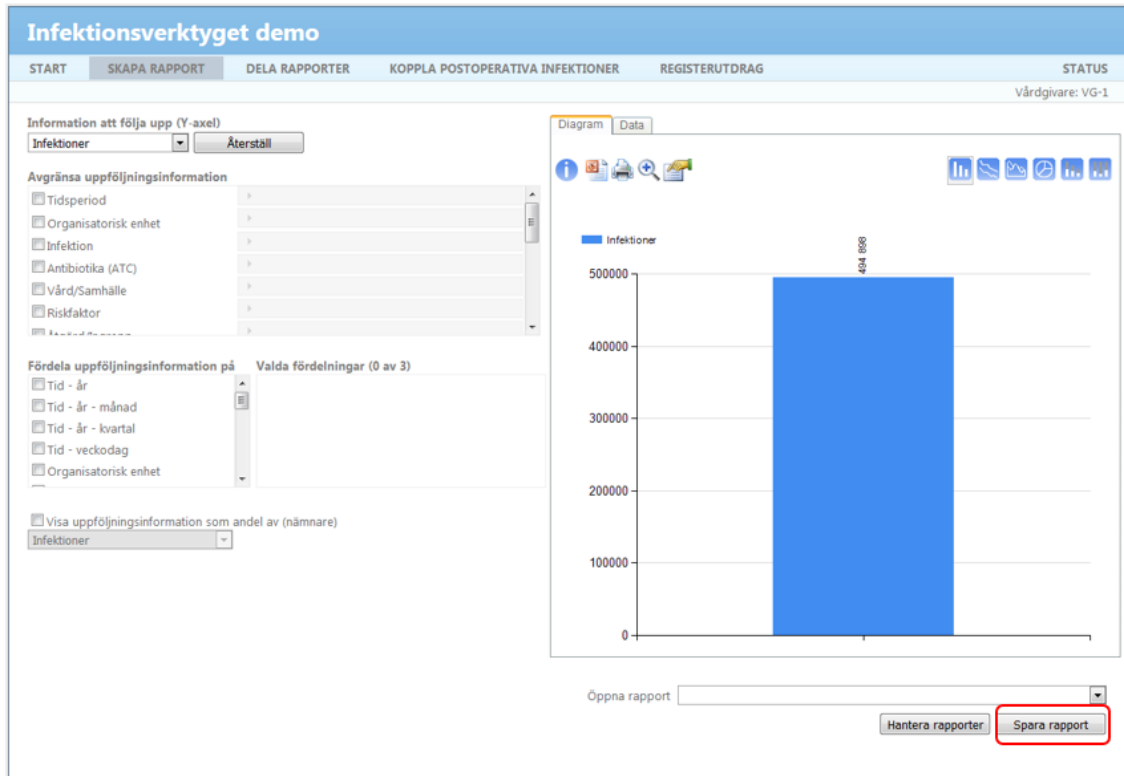
Figur 9 Spara rapport.
